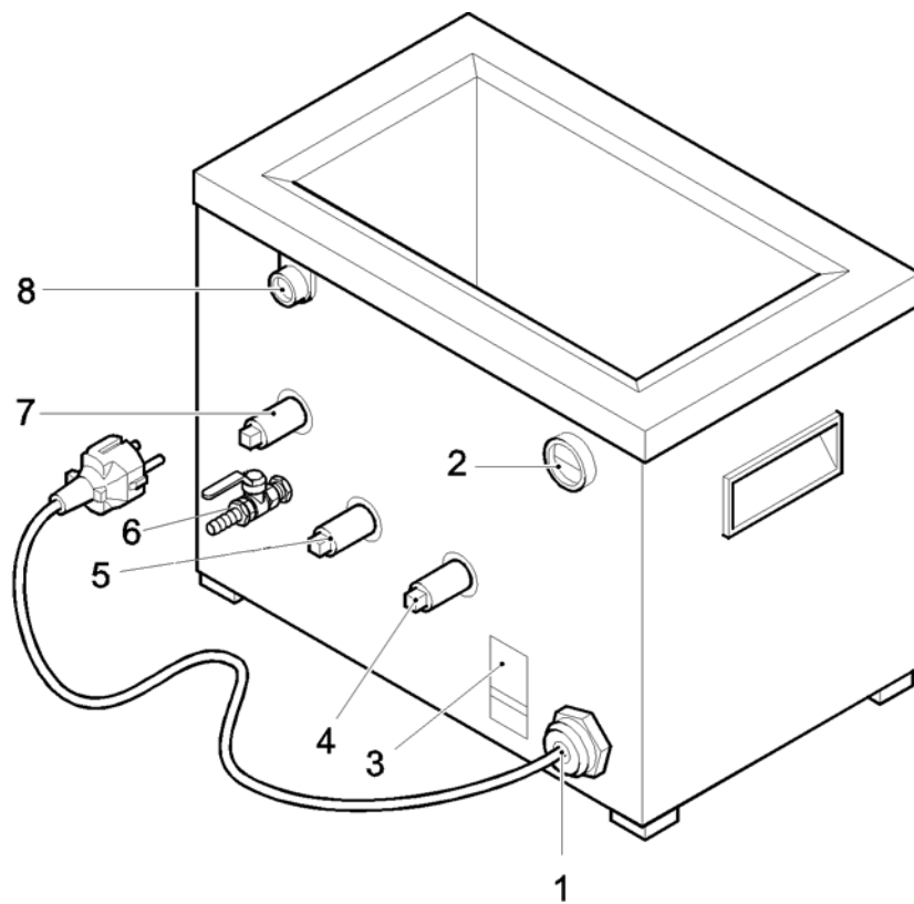
Bild 5.2 Geräterückseite
