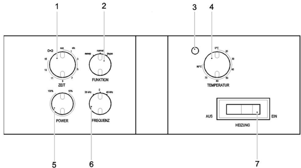
Bild 7.1 Bedienelemente Gerätevorderseite
