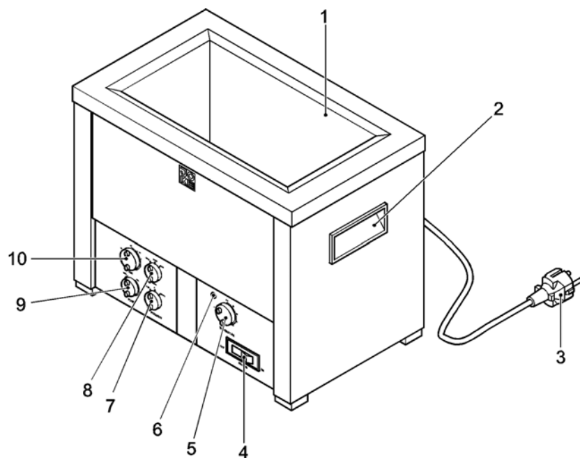
Bild 5.1 Gerätevorderseite
